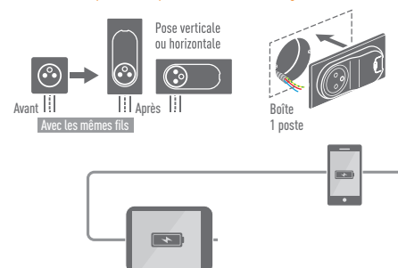
Prise de courant Surface + chargeur USB (s'installe à la place d'une prise existante sans changer la boîte)
