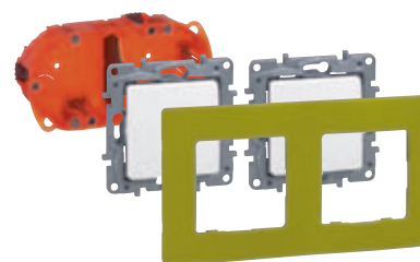
Montage dans boîte 2 ou 3 postes, en horizontal ou en vertical
